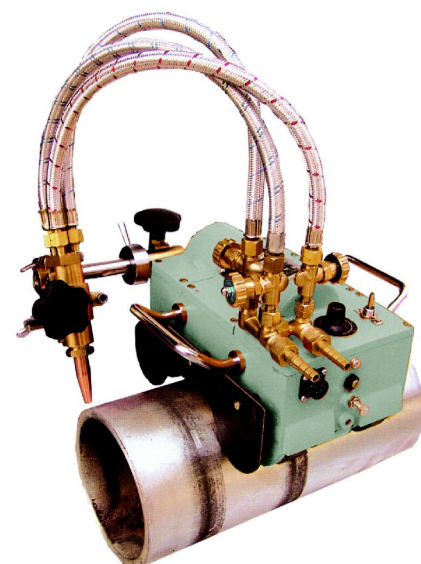
Skjæremaskin Magnet ZCM-11
