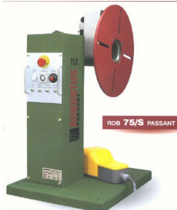
Dreieplate med gjennomgående hull opp til 200mm (rørgjennomgang)
